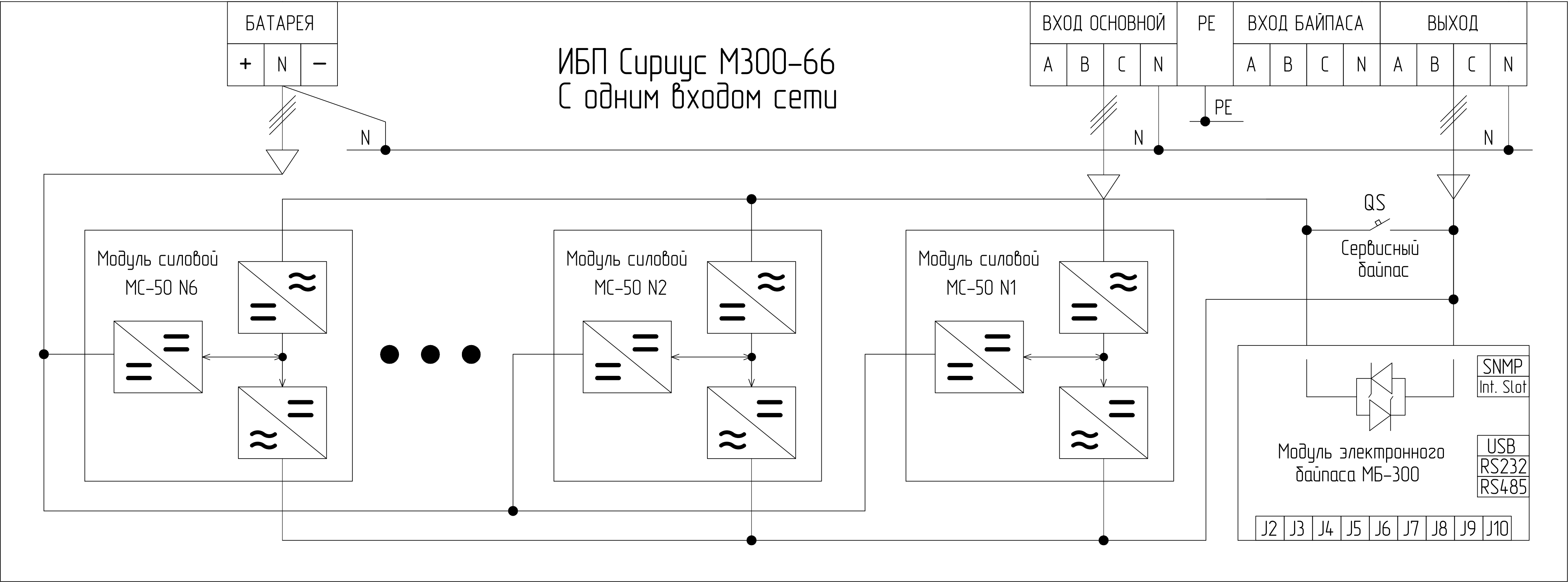
Схема с одним входом сети (Вход байпаса не используется)
