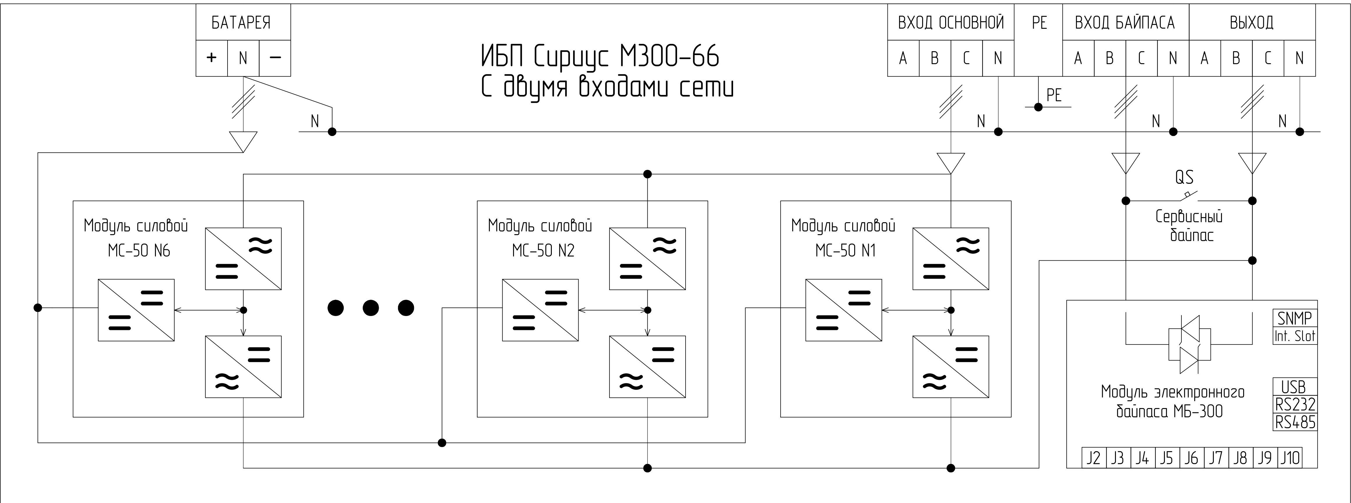
Схема с двумя входами сети (Вход основной и Вход байпаса)
